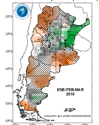
Pronóstico de Precipitación (Modelo 2)
