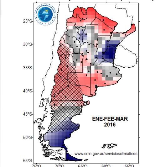
Pronóstico de Temperatura Media (Modelo 2)
