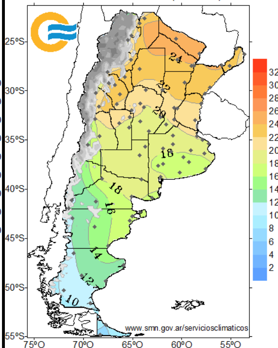
TEMPERATURA MEDIA (°C) FEBRERO-MARZO-ABRIL (1981-2010)
